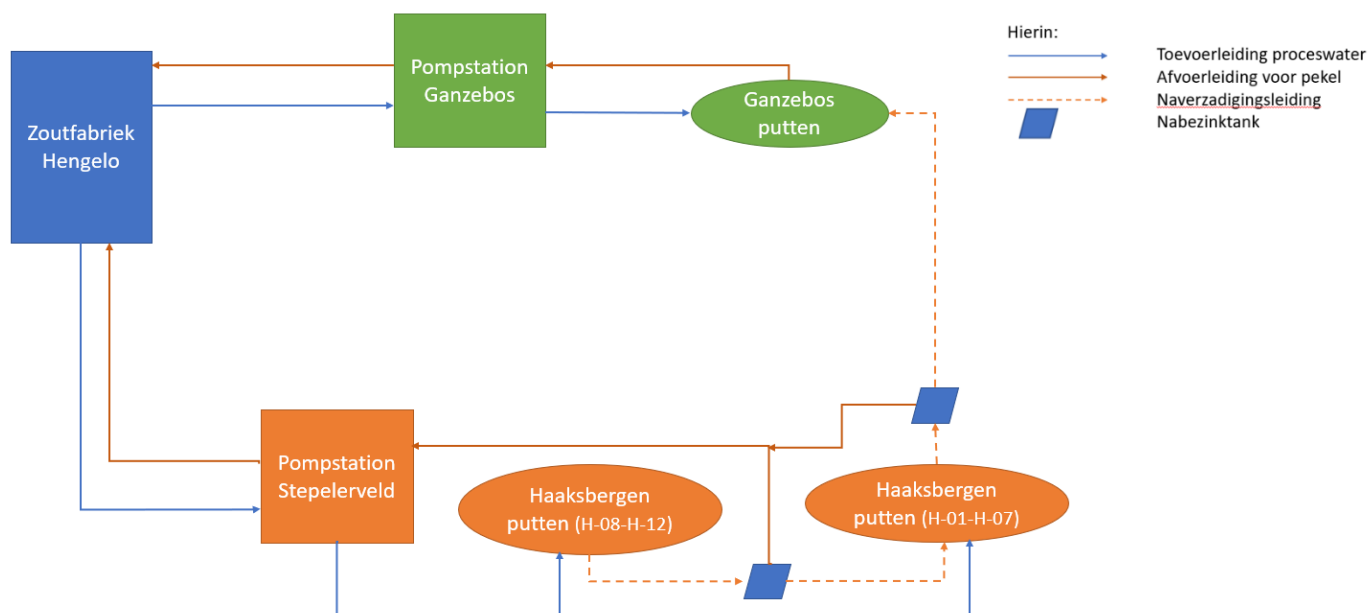
Afbeelding 3: Schematische weergave van de diverse (water)stromen
