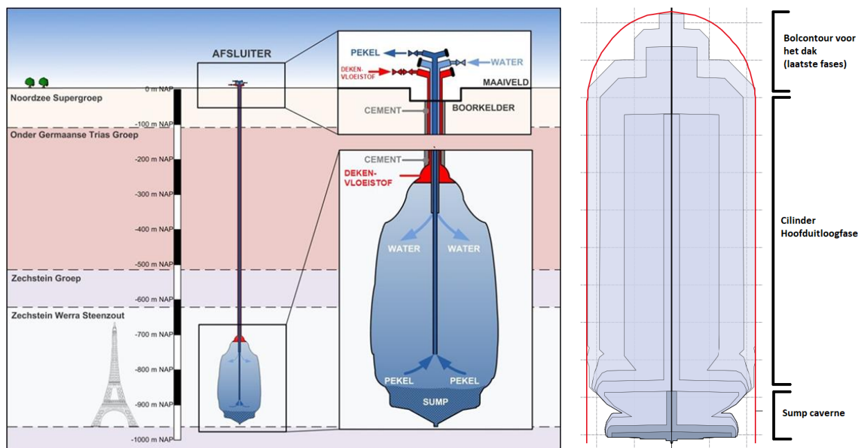
Afbeelding 4: Links: Schematische weergave zoutwinning middels oplosmijnbouw. Rechts: Schematische opbouw van de verschillende uitloingsstappen van een cave'ne binnen de maximale uitloingscontour (rode lijn).
